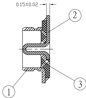
SECT A-A"
