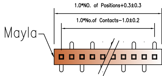
A TYPE FH-1.0-1019-xx03N
