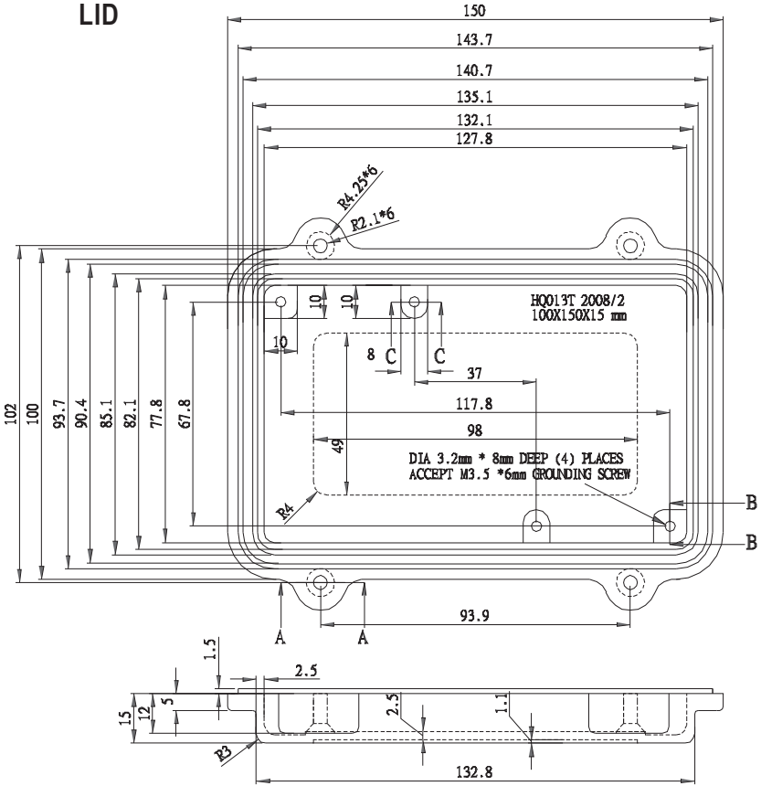
DETAIL A-A
