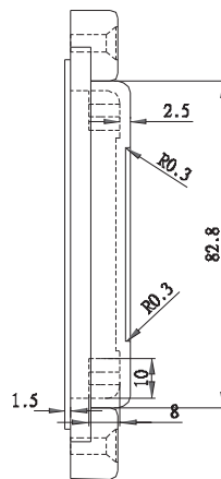
DETAIL A-A
