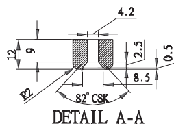
DETAIL A-A
