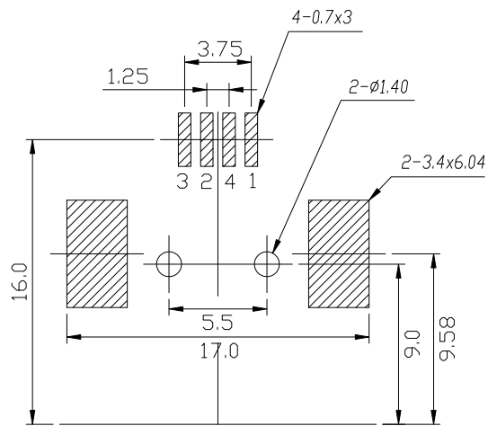
PCB EDGE PCB LAYOUT (COMPONENT SIDE)
