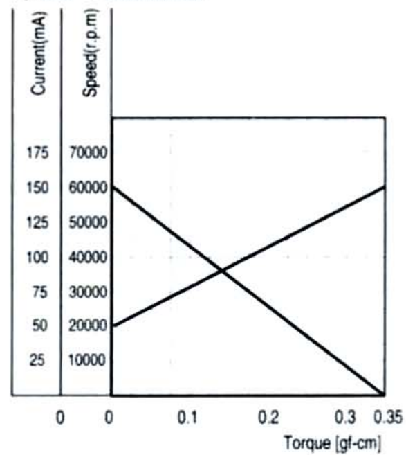
特性图 Characteristics
