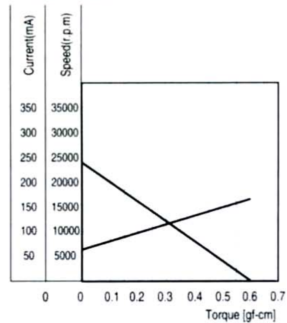
特性图 Characteristics
