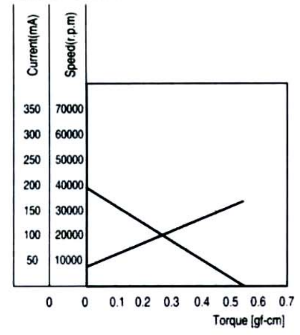
特性图 Characteristics
