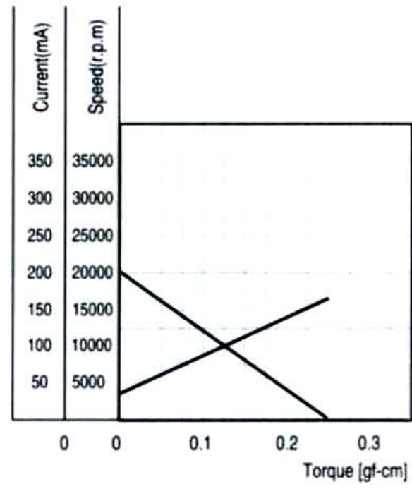
特性图 Characteristics
