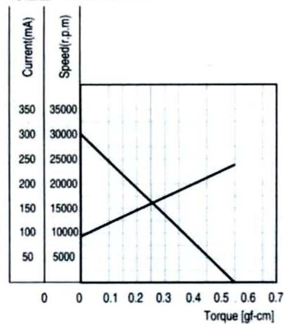
特性图 Characteristics
